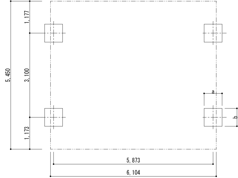
■ 基礎配置図
